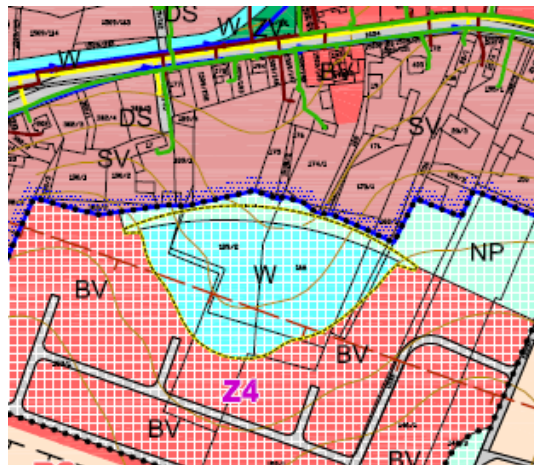
Výřez z Koordinačního výkresu
