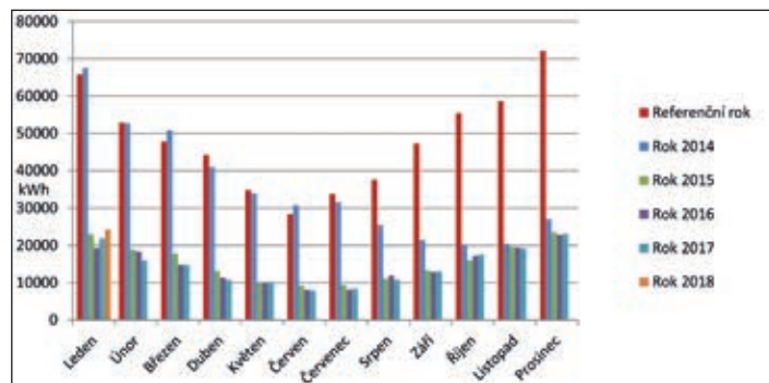
pozn. Graf měsíčních spotřeb EE na veřejném osvětlení města Holice. Výměna za LED svítidla proběhla od června do září 2014
